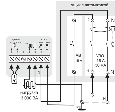
Схема 2. Подключение автоматического выключателя и УЗО вертикали с шириной жала не более 3 мм. Отвертка с жалом шириной более 3 мм может нанести механические повреждения клеммам. Это может повлечь потерю права на гарантийное обслуживание. Затягивать клеммы необходимо с моментом не более 0,5 Н × м.
