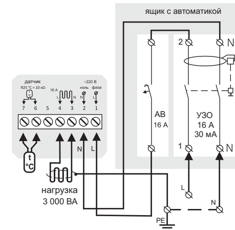
Схема 2. Подключение автоматического выключателя и УЗО вертикали с шириной жала не более 3 мм. Отвертка с жалом шириной более 3 мм может нанести механические повреждения клеммам. Это может повлечь потерю права на гарантийное обслуживание. Затягивать клеммы необходимо с моментом не более 0,5 Н × м.
