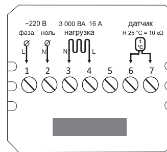
Схема 1. Схема подключения и упрощенная внутренняя схема
